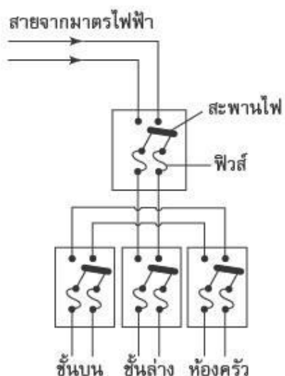
รูปที่ 1 แสดงตัวอย่างวงจรไฟฟ้าในบ้าน
